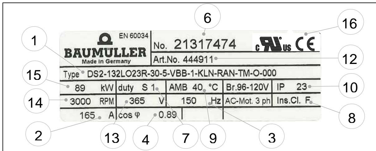
Bild 2: Typenschild Baugröße 100-132
