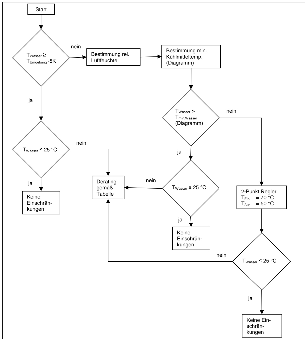
Bild 9: Funktionsschema Kühlmiteleintrittstemperatur
