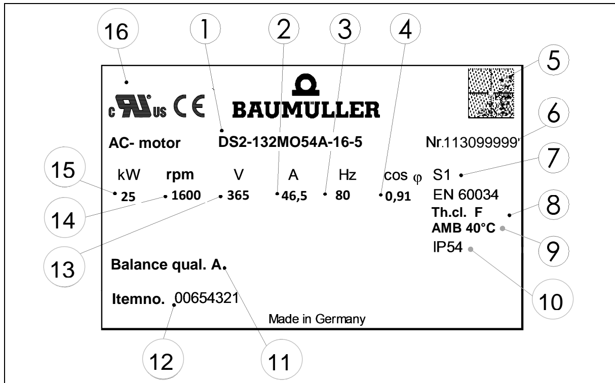
Bild 1: Typenschild Baugröße 160-200
