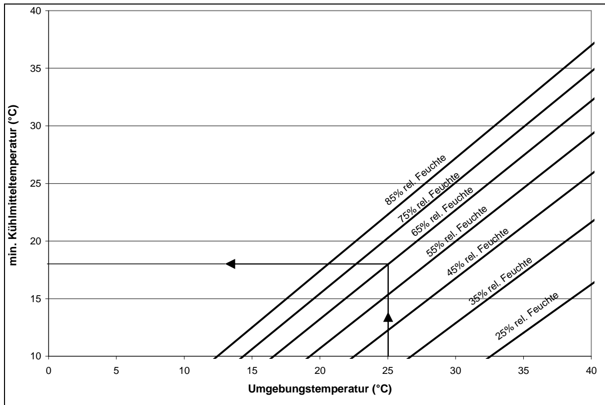
Bild 8: Ermittlung der Kühlmitteltemperatur
