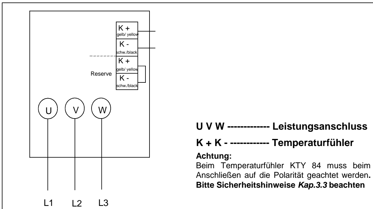
Bild 3: Hauptanschluss mit Klemmenkasten
