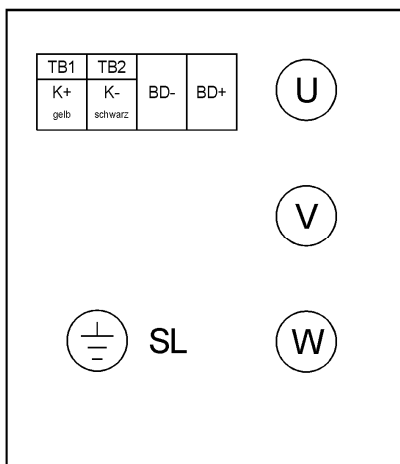
Bild 3: Klemmenbelegung mit Temperatursensor und Bremse
