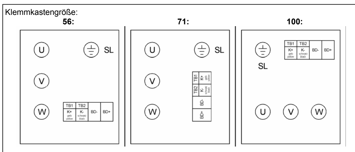
Bild 4: Klemmenbelegung Sondervariante
