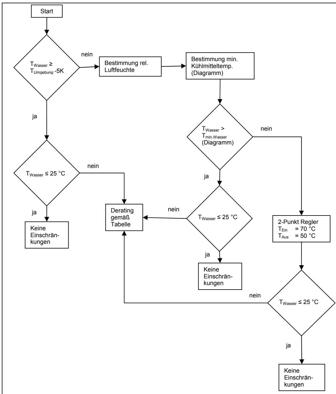
Bild 13: Funktionsschema Kühlmittleintrittstemperatur
