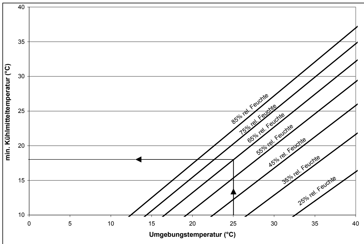
Bild 12: Ermittlung der Kühlmitteltemperatur
