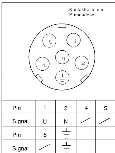
Bild 6: Polbelegung Lüfteranschluss
