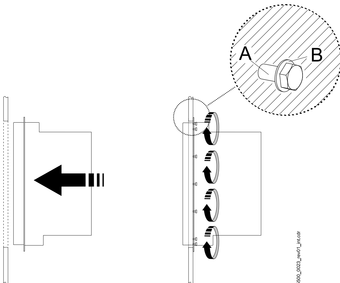
Abbildung 76: Mounting instruction „diverse“
